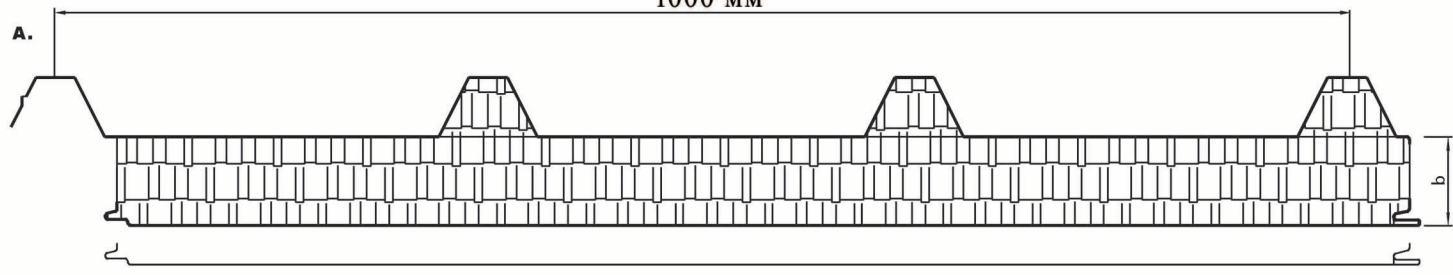
Замок 8*A: Z-lock. Кровельная панель
