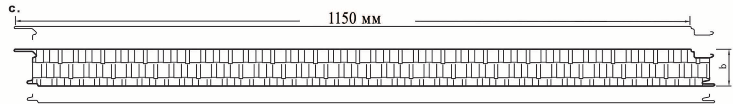
Замок 8*C потайной: Z-lock. Стеновая панель
