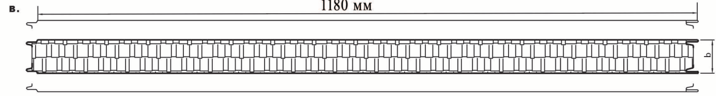
Замок 8*C потайной: Z-lock. Стеновая панель
